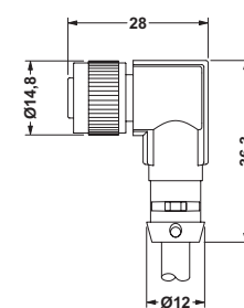
Hona M 12 x 1, vinklat utförande med LED
