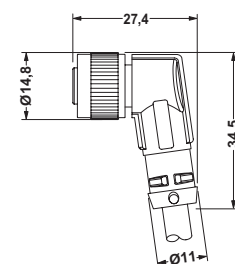
Hona M 12 x 1, vinklat utförande
