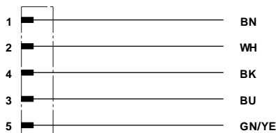
Anslutna M 12-kontakter
